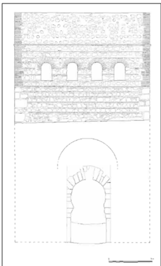
Alzado principal de la Puerta del Vado. Fuente: La Puerta del Vado de Toledo . Arturo Ruiz Taboada y Jacobo Fernández del Cerro, 2009.
